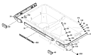
ETB-0000001178, Oświetlenie z żarówkami do rocznika model. 2020 włącznie
