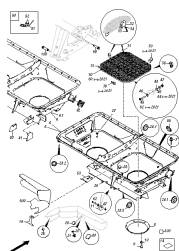
ETB-001359, Rama i zbiornik ZA Super / Ultra / Special
