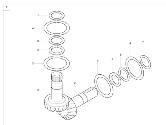
ETB-001398, Zestaw naprawczy do wałków przekładni 8 kW
