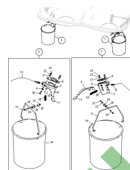
ETB-001438, Urządzenie do ustawiania odpowiedniej dawki rozsiewu
