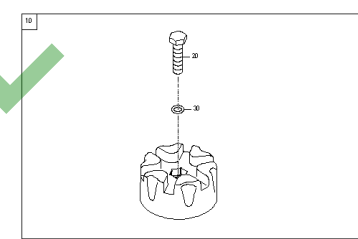
ETB-0000010880, Śruba centralna
