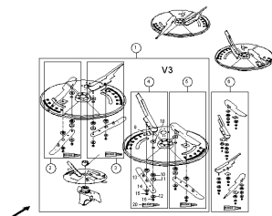
ETB-001390, Zestaw łopatek rozsiewających V3
