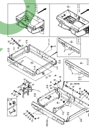
ETB-001367, Nadstawka przykręcana
