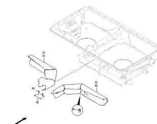
ETB-001065, Osłona przeciwbryzgowa jednoczęściowa
