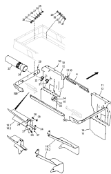
ETB-001085, Belka oświetlenia / osłona przeciwbłotna
