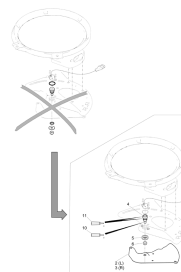
ETB-001382, Zestaw do przeosażenia dna z otworami ZA-V do nr masz. ZA00001050
