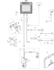
ETB-001154, Zestaw do konwersji komputera podstawowego ZA-V / ZA-TS Hydro
