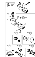
ETB-0000011658, Skrzynia biegów na zewnątrz Hydro Lewa od ZA00039421
