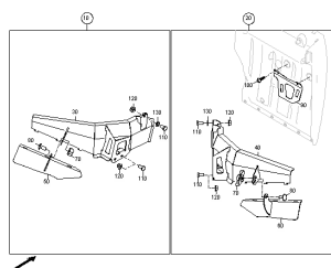
ETB-0000000937, Ekran rozsiewu granicznego prawy
