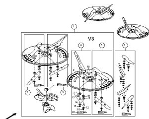
ETB-001390, Zestaw łopatek rozszewających V3
