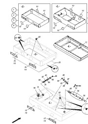
ETB-001366, Nadstawka spawana
