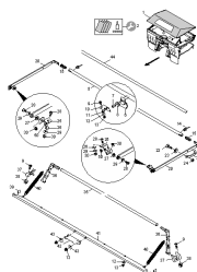
ETB-001429, Składana plandeka S
