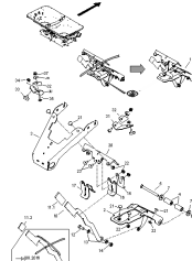
ETB-001439, Konsola ekranu rozsiewu ręczna
