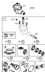
ETB-001394, Przekładnia zewnętrzna 12 kW - EA343
