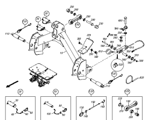
ETB-0000005125, Rama nakładkowa Ultra Quickhitsch
