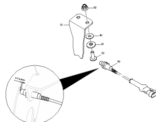
ETB-0000012320, Czujnik do sygnalizacji położenia dyfuzora
