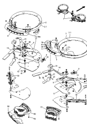
ETB-001384, Dno z otworami ZA-V hydrauliczne
