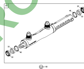
ETB-0000012454, Siłownik hydrauliczny D 18-16-80-277
