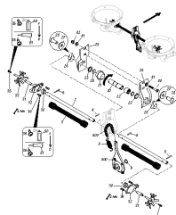
ETB-001380, Wałek mieszadła ZA- V
