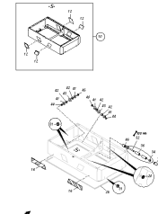
ETB-001365, Nadstawka S 2600 spawana
