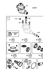
ETB-001394, Przekładnia zewnętrzna 12 kW - EA343
