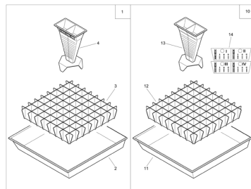
ETB-001431, Ruchome stanowisko pomiarowe
