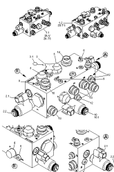
ETB-001404, Blok sterowania
