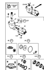
ETB-0000011656, Skrzynia biegów na zewnątrz Hydro Left to ZA00039420
