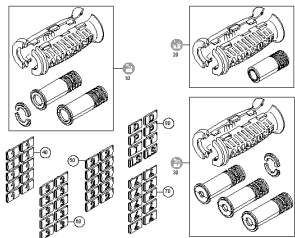
ETB-001386, Uchwyt węży hydraulicznego
