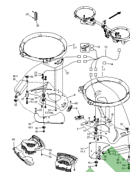
ETB-001383, Dno z otworami ZA-V Easy i Control
