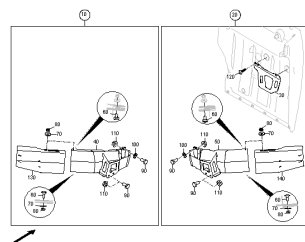
ETB-0000000930, Ekran rozsiewu zagonowego
