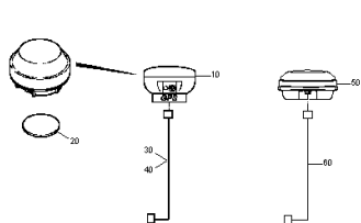
ETB-001418, Odbiornik GPS
