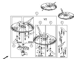
ETB-001389, Zestaw łopatek rozsywających V2
