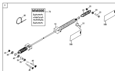
ETB-001436, Wskaźnik pozycji ekranu rozsiewu/limitera
