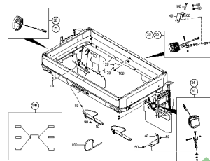
ETB-003484, Zestaw oświetlenia roboczego
