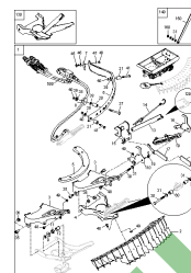
ETB-001434, Limiter V prawy
