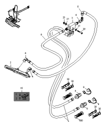
ETB-001435, Hydraulika limiterów
