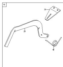
ETB-0000009517, Zestaw modernizacyjny man. Wspornik dyfuzora
