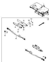
ETB-001378, Zestaw oświetleniowy do rozświeczacza przedniego
