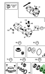
ETB-0000011657, Skrzynia biegów na zewnątrz Hydro Prosto z ZA00039421
