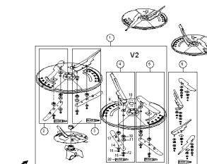
ETB-001389, Zestaw łopatek rozsiewających V2
