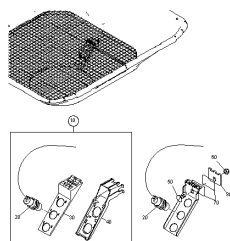
ETB-001416, Czujnik stanu naładowania
