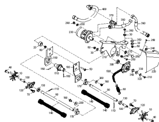
ETB-0000010882, Mieszadło ZA-V Hydro
