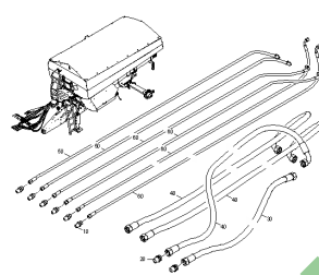
ETB-0000010241, Wiązka uchwytu USA/Kanada
