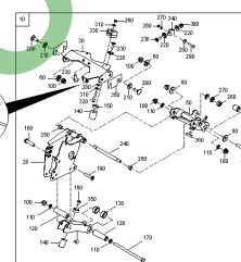
ETB-0000000840, Wspornik dyfuzora hydrauliczny (1)
