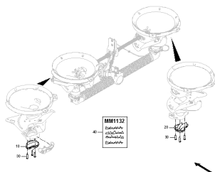
ETB-0000007019, Zestaw do rozsiewania boczny
