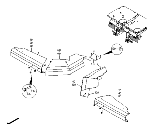
ETB-001066, Osłona przeciwbryzgowa dwuczęściowa
