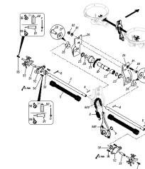
ETB-001380, Wałek mieszadła ZA-V
