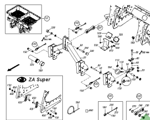
ETB-0000001627, ZA Super Profis (2)
