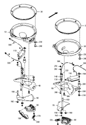
ETB-0000005380, Zestaw podłogowy ZA-V Control 2
