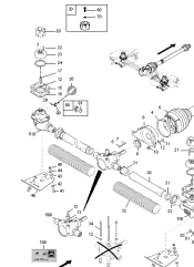
ETB-001391, Napęd V mechaniczny
