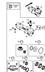
ETB-0000011657, Skrzynia biegów na zewnątrz Hydro Prosto z ZA00039421
