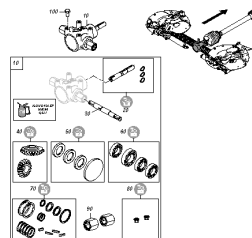
ETB-0000010477, Skrzynia biegów w połowie 11KW
