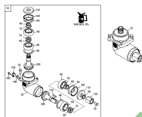
ETB-001395, Przekładnia zewnętrzna 8 kW
