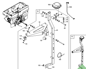
ETB-0000006206, Uchwyt na odbiornik GPS
