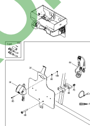
ETB-001377, Uchwyt tablicy rejestracyjnej
