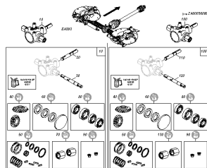
ETB-001393, Przekładnia środkowa 11 kW
