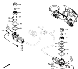
ETB-001399, Mechanizm rozsiewający ZA-V Hydro
