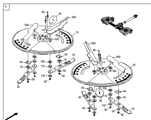
ETB-0000011797, Zestaw dyfuzora V3
