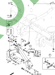
ETB-001358, ZA-Ultra bez techniki ważenia
