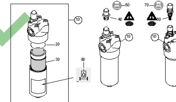
ETB-006791, Filtr hydrauliczny ciśnieniowy
