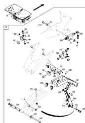
ETB-001440, Wspornik dyfuzora hydrauliczny (1)
