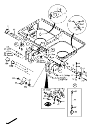
ETB-001362, Elementy ramowe
