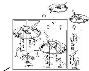
ETB-001388, Zestaw łopatek rozsiewających V1
