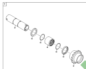
ETB-0000010883, Wolnobieg tulei
