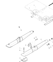
ETB-001428, Plandeka zwijana S i L hydrauliczna
