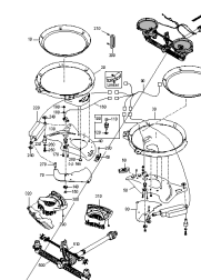
ETB-0000001650, Dno z otworami ZA-V Easy 2
