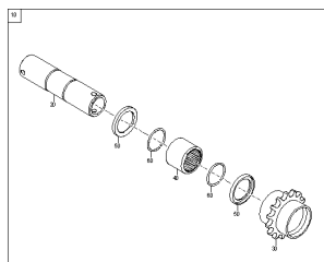
ETB-0000010883, Wolnobieg tulei
